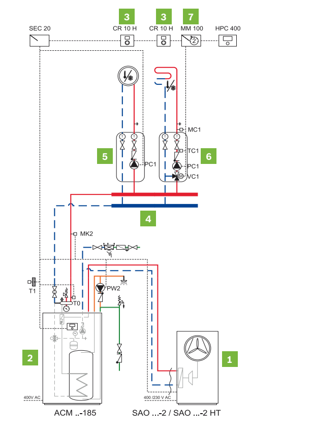
Esquema de instalación ACM (acumulación)
