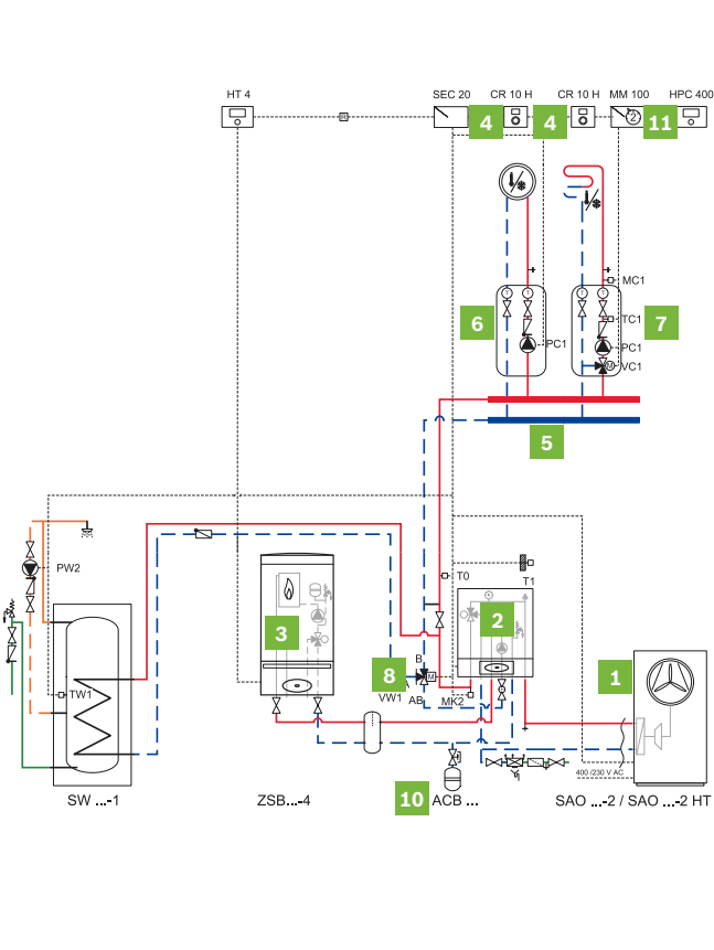
Esquema de instalación ACB (híbrida)
