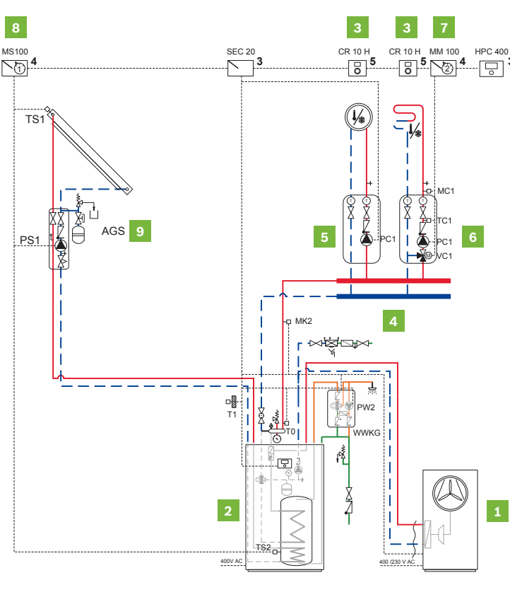
Esquema de instalación ACMS (acumulación solar)
